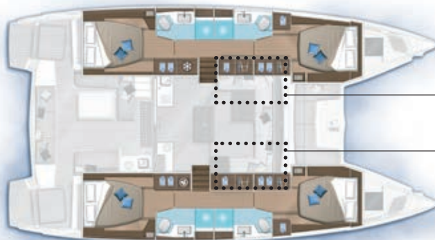
4 cabines, 4 salles d'eau / 4 cabins, 4 bathrooms
